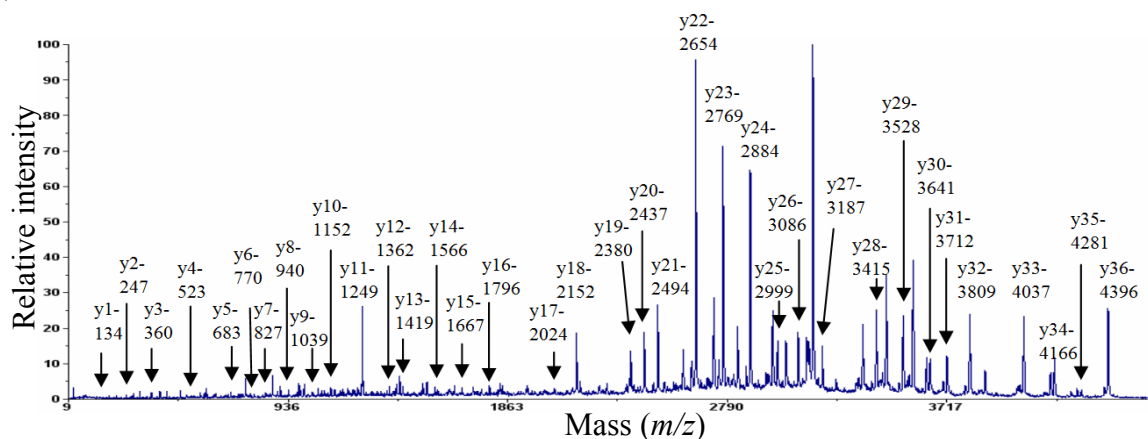
Figure 41. MS/MS spectra of double S-tagged morintide C2. C NEM : S-NEM cysteine; C IAA : S-IAA cysteine. A) MS/MS spectra of 4261-Da peptide showed a C NEM -C IAA -C IAA -C NEM -C IAA -C IAA alkylation pattern, establishing the Cys I-IV connectivity; B) MS/MS data of 4397-Da peptide showed a C NEM -C NEM -C IAA -C NEM -C NEM -C IAA alkylation pattern establishing the Cys III-VI connectivity; C) MS/MS data of 4397-Da peptide showed a C NEM -C IAA -C NEM -C NEM -C IAA -C NEM alkylation pattern establishing the Cys II-V connectivity.
